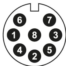
Вилка M16 (вид со стороны датчика)
