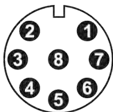
Вилка M12-A (вид со стороны датчика)
